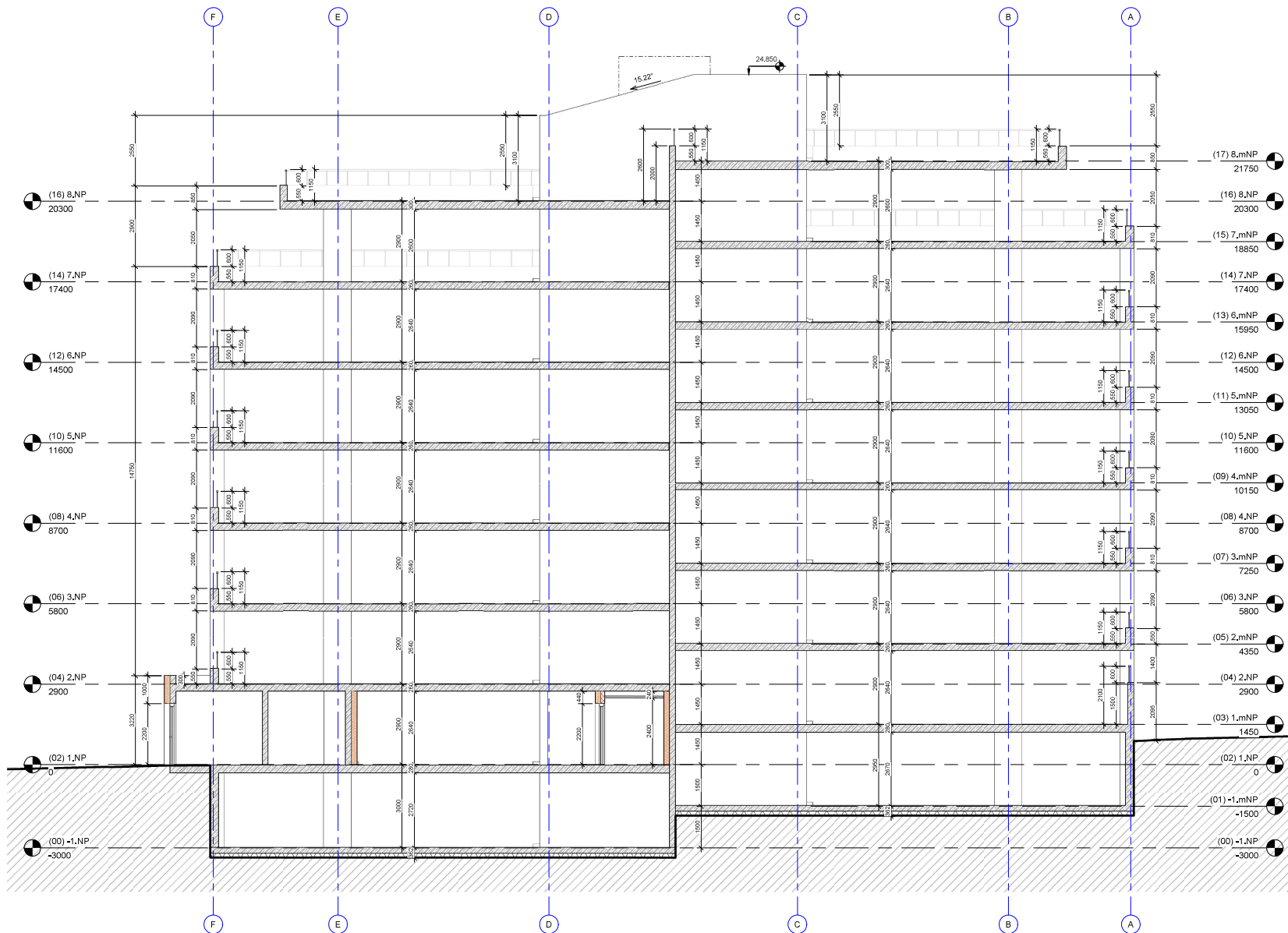
1 Řez C-C' 1 : 75
